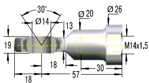
E14-VA Swivel Eye
