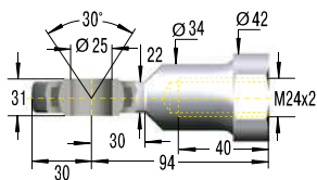
E24 Swivel Eye DIN 648
