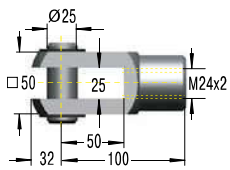
D24 Clevis Fork DIN 71752
