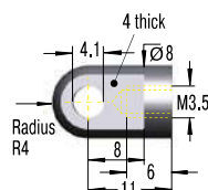
A3,5-V4A Eye
