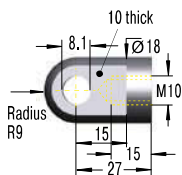
A10-VA Eye
