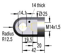
A14-VA Eye
