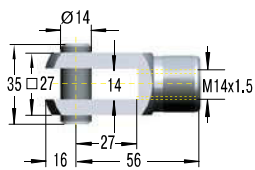
D14-VA Clevis Fork
