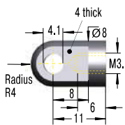
A3,5-V4A Eye
