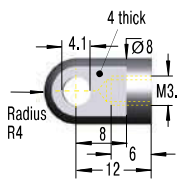
A3,5 Eye
