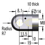
A8-VA Eye
