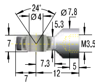
E3,5 Swivel Eye DIN 648
