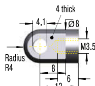
A3,5 Eye
